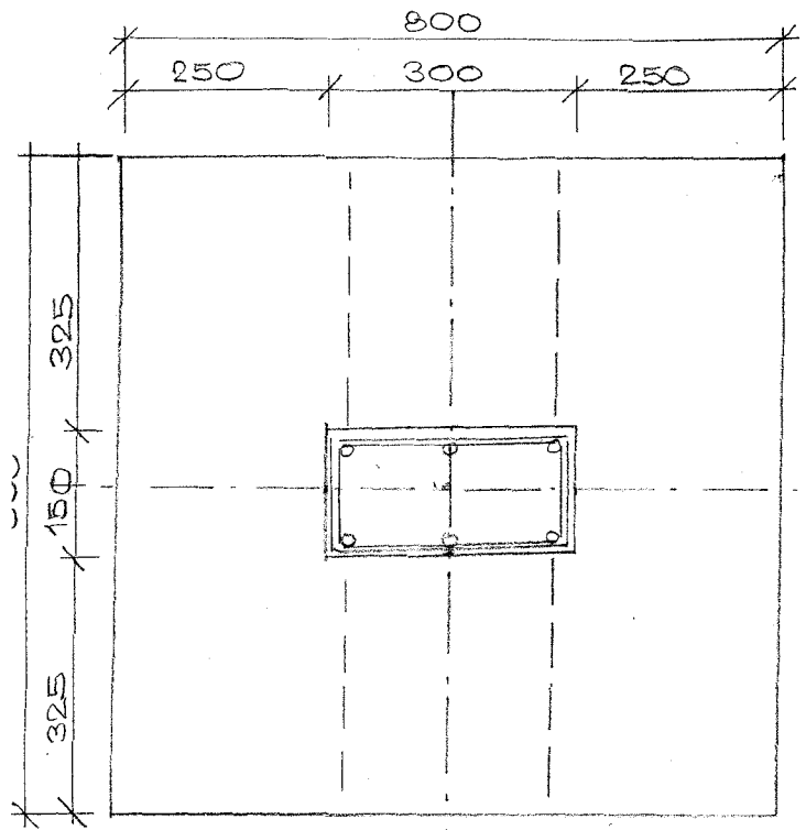
PŮDORYS
