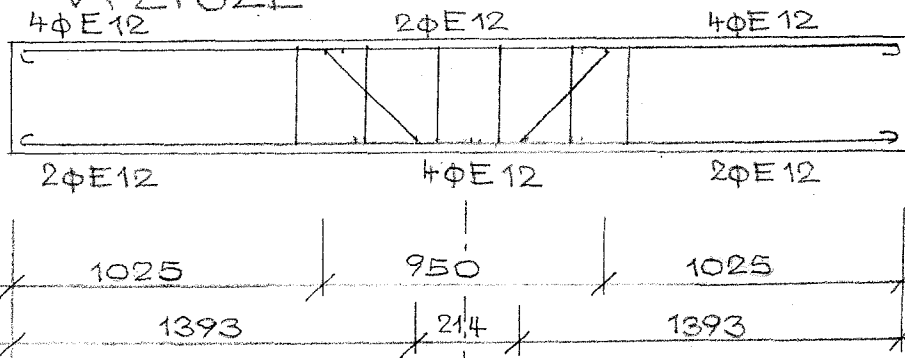
VÝKRES VÝZTUŽE
