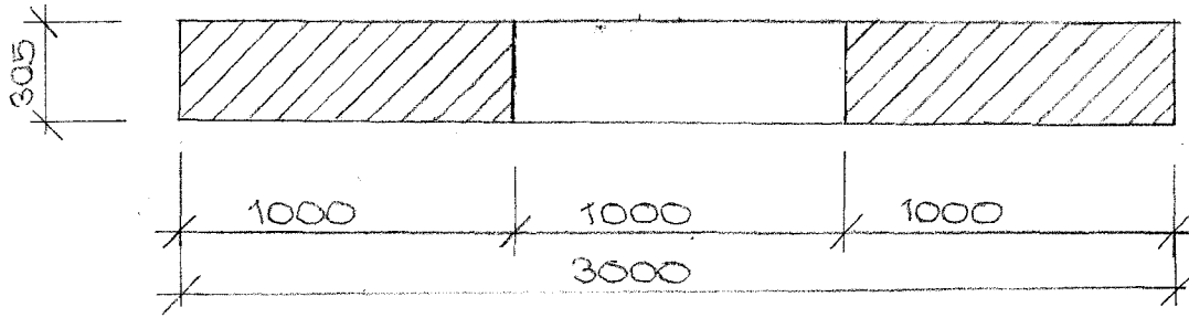
NÁRYS
